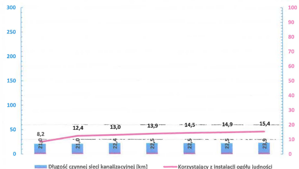
Wykres 7. Długość sieci kanalizacyjnej oraz wskaźnik skanalizowania gminy Żabia Wola w latach 2016 – 2022 Źródło: opracowanie własne na podstawie danych GUS oraz danych Urzędu Gminy
